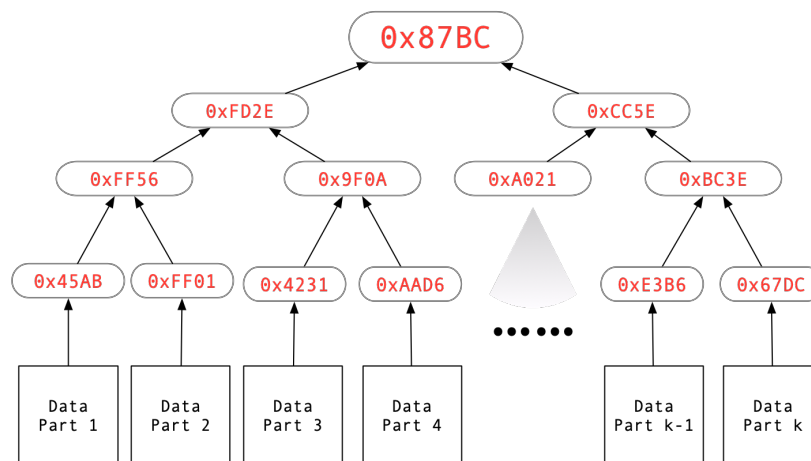
Racine de l'arbre Merkle
