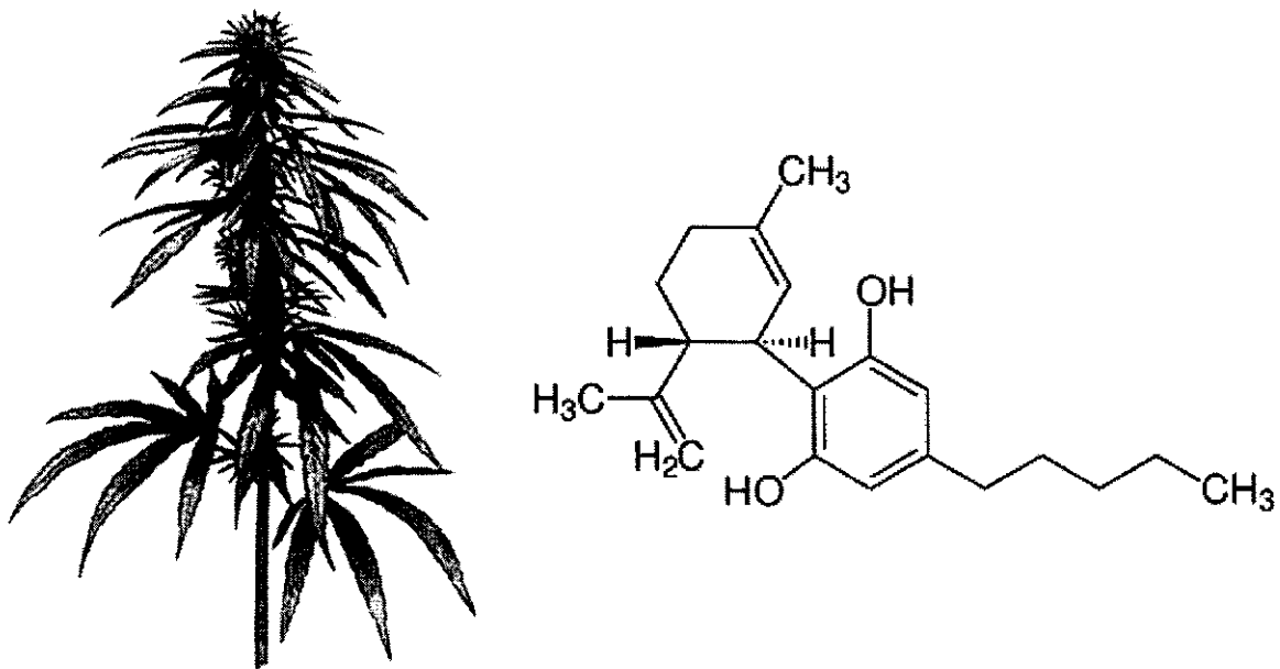
Figure 4. Structure moléculaire du cannabidiol extrait du Cannabis sativa L..
