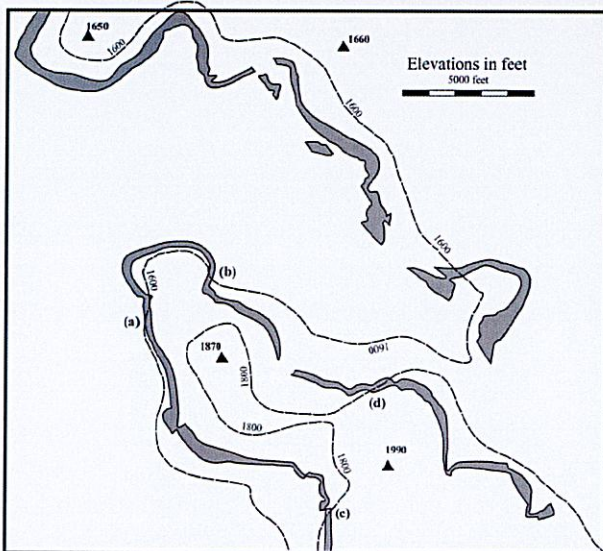
Affleurement de la « Firestone Sandstone Formation » (Alston map, northern England)
